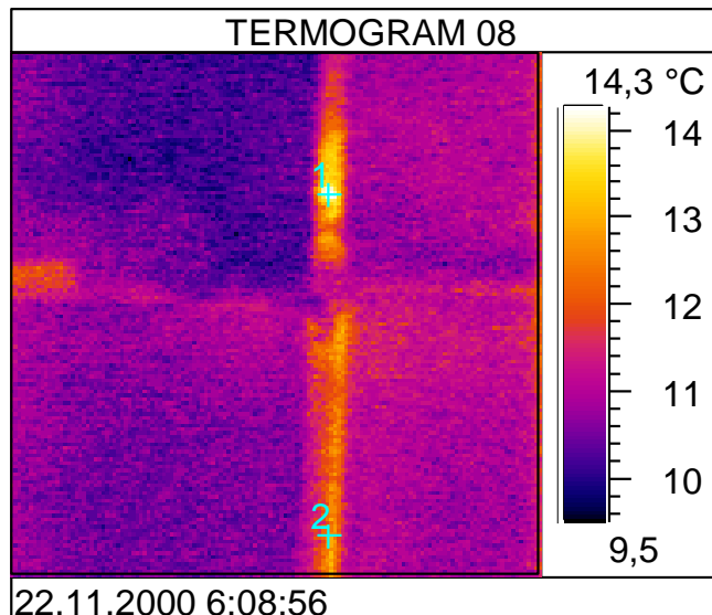
▲ Tepelnoizolačná nehomogenita v oblasti stykov na západnom štíte Thermoinsulation inhomogeneity in the place of joints on the west
